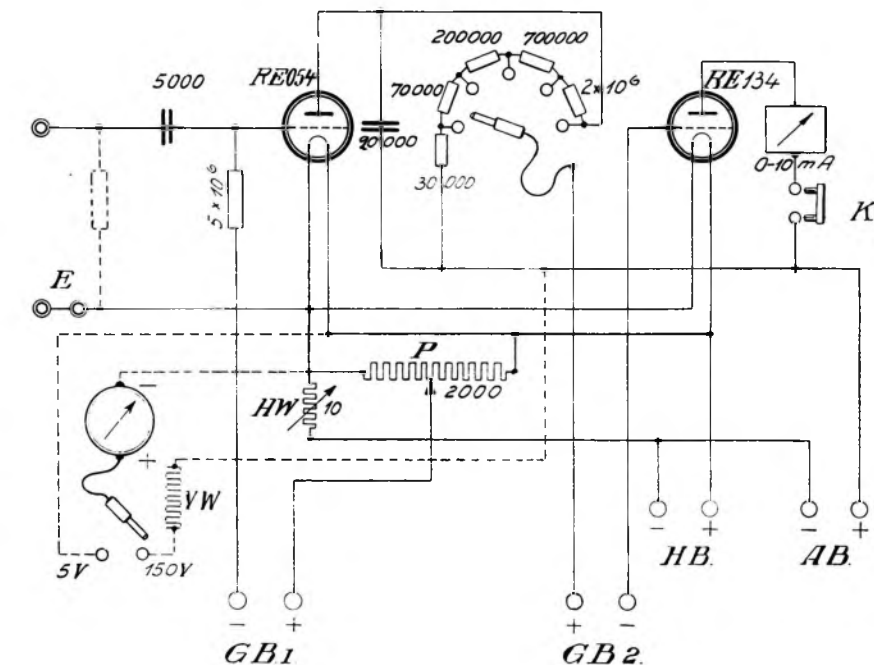
Fig. 1. E = Aarde HW = Gloeiweerstand P = Potentiometer
